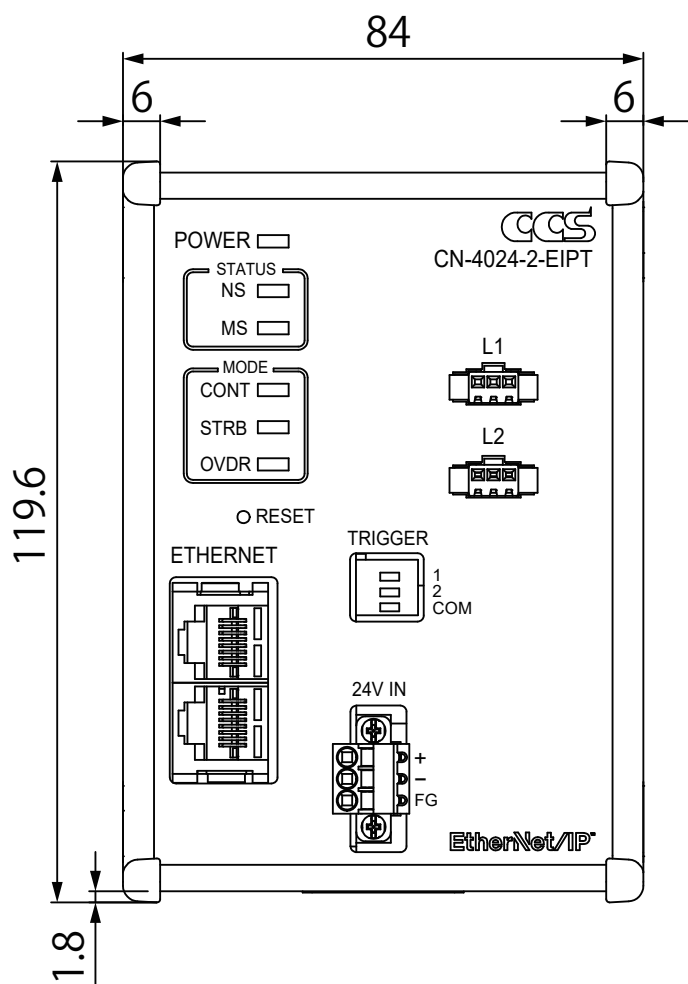
天面
