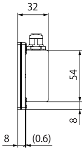
【側面】
