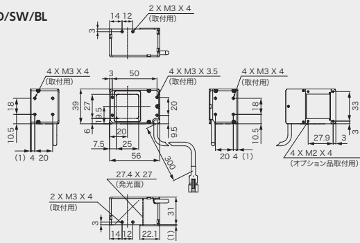
LFV3-G-35RD/SW/BL
