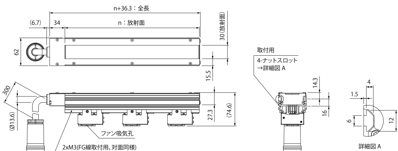
LNSP-□□□UV365-FNNR(ワイドタイプ)
