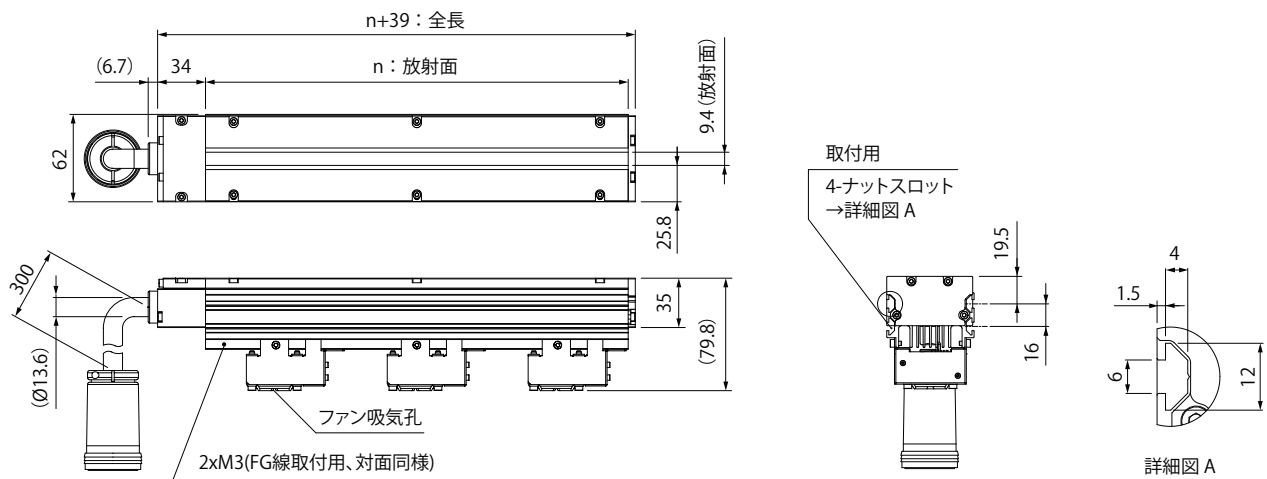
LNSP-□□□UV365-FN(ナロータイプ)
