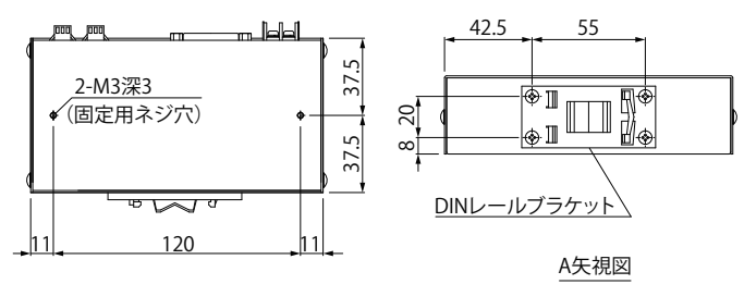
A矢视图
