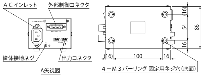
A矢视图
