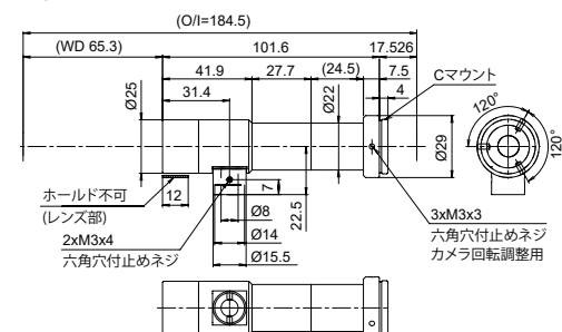
SE-65VT40-M
