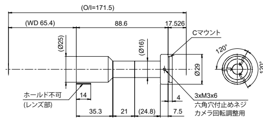
SE-65ST20-M
