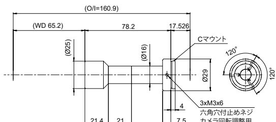
SE-65ST60-M
