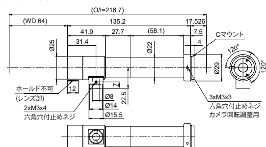
SE-65VT60-M
