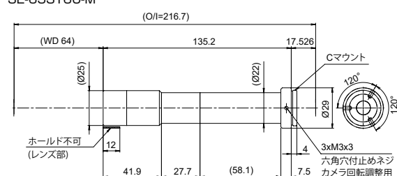
SE-65ST60-M
