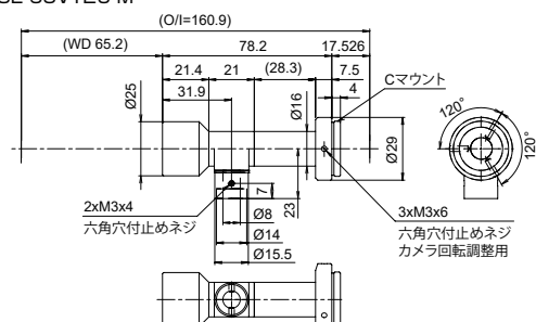
SE-65VT20-M
