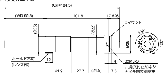
SE-65ST40-M
