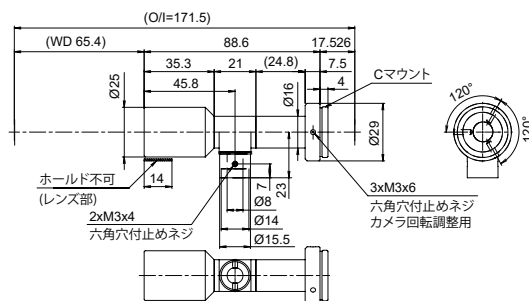
SE-65VT20-M
