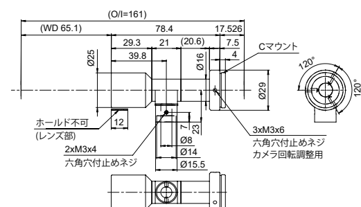
SE-65VT40-M
