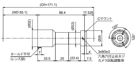
SE-65ST10-M
