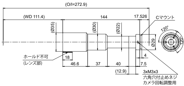
SE-110ST30-M
