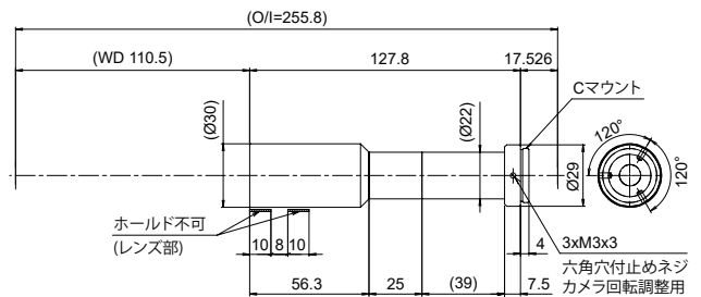
SE-110ST20-M
