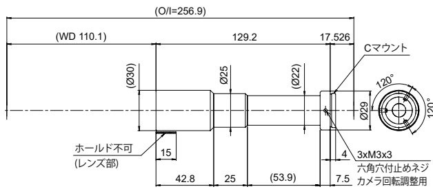
SE-110ST30-M
