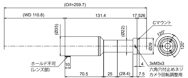
SE-110ST10-M
